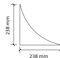
Circle end E1 238 x 238 mm
