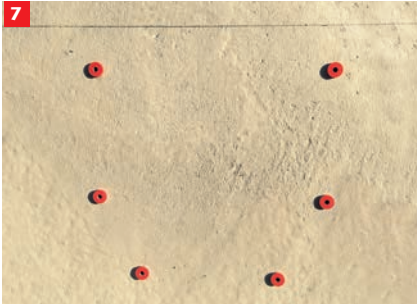
7 Obere Bohrungen setzen und Dübel mit Distanzscheibe einstecken
