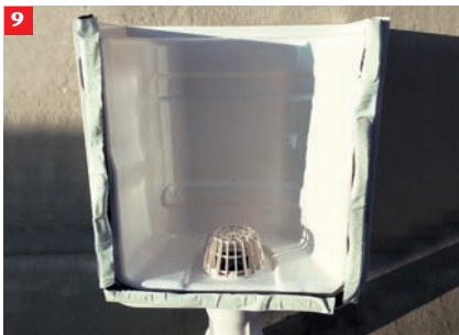
9 Dichtungsband aufkleben und Schutzfolie entfernen. Befestigungspunkte vollständig überkleben
