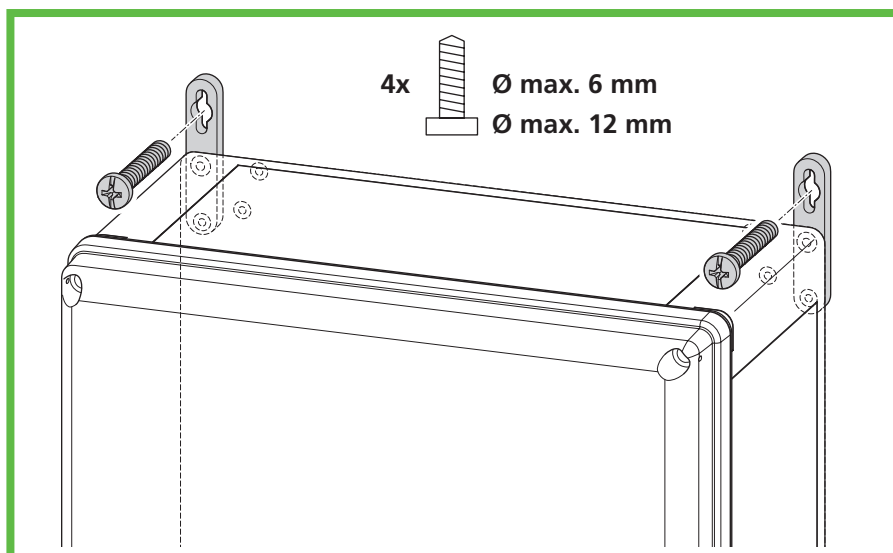
Abb. 45: Wandmontage
