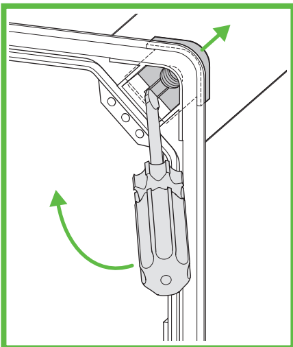
Abb. 51: Demontage Gewindeinschübe GEOS 3030, GEOS 3040 GEOS 4050
