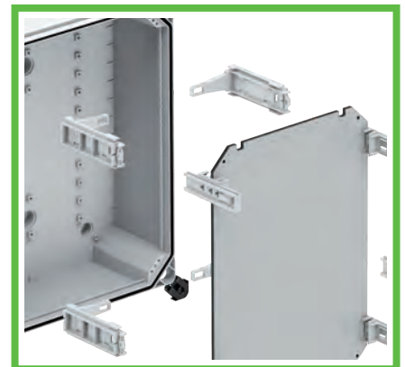
Abb. 13: Systemaufbau Montagesystem
