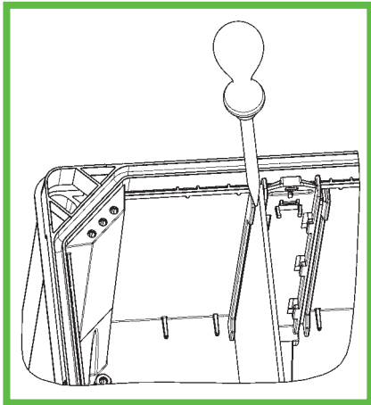
Abb. 80: Demontage Trennwand
