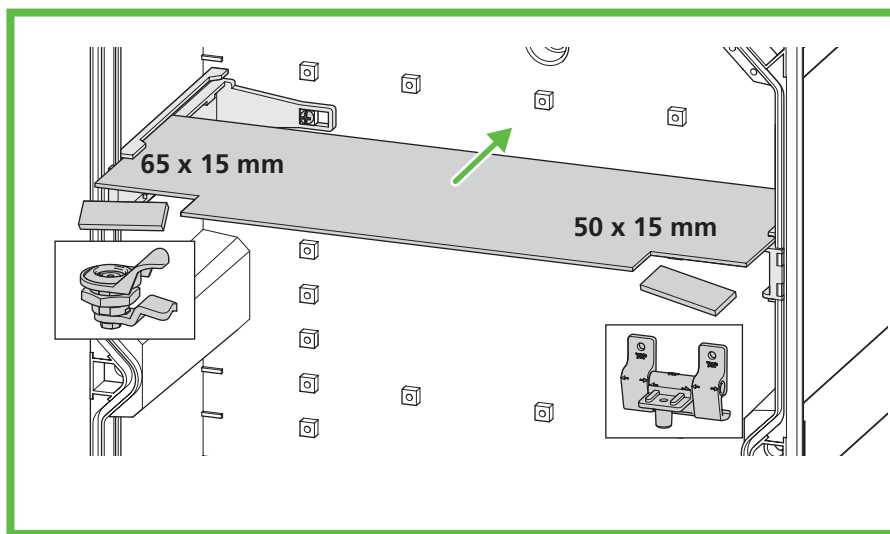
Abb. 84: Aussparungen sägen
