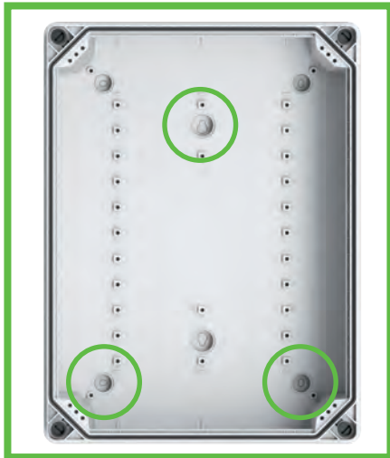
Abb. 41: Befestigungspunkte 3-Punkt-Montage
