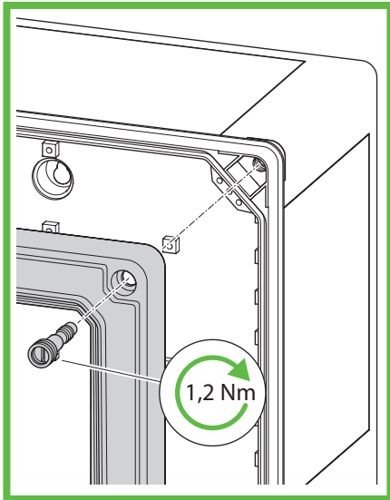
Abb. 57: Montage Schnellgewindeschraube
