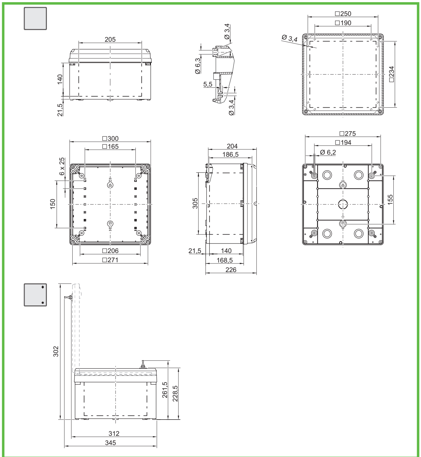
Abb. 91: GEOS 3030-22
