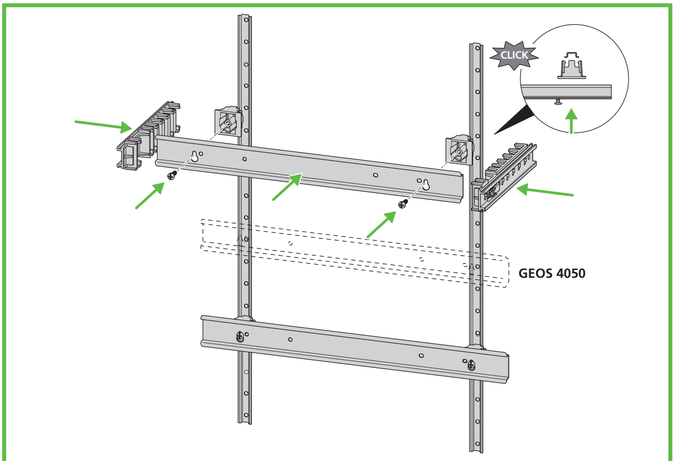
Abb. 75: Montage Traggestell
