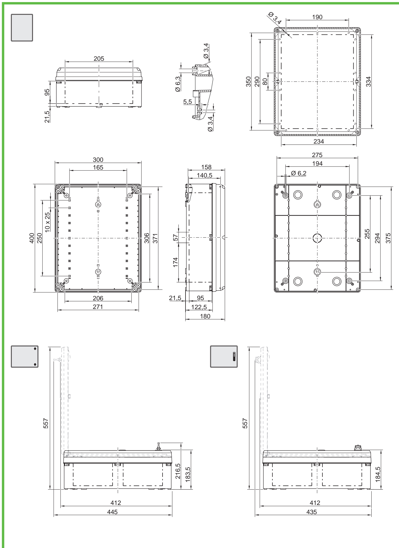
Abb. 94: GEOS-S 4030-18
