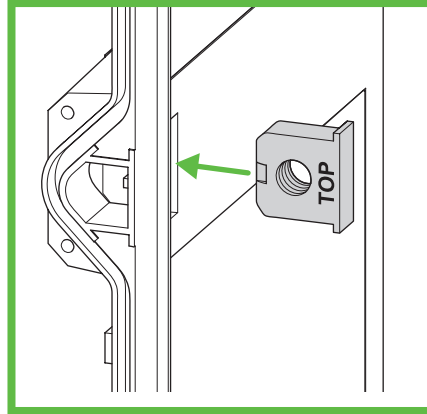
Abb. 50: Montage Gewindeinschübe GEOS 4050
