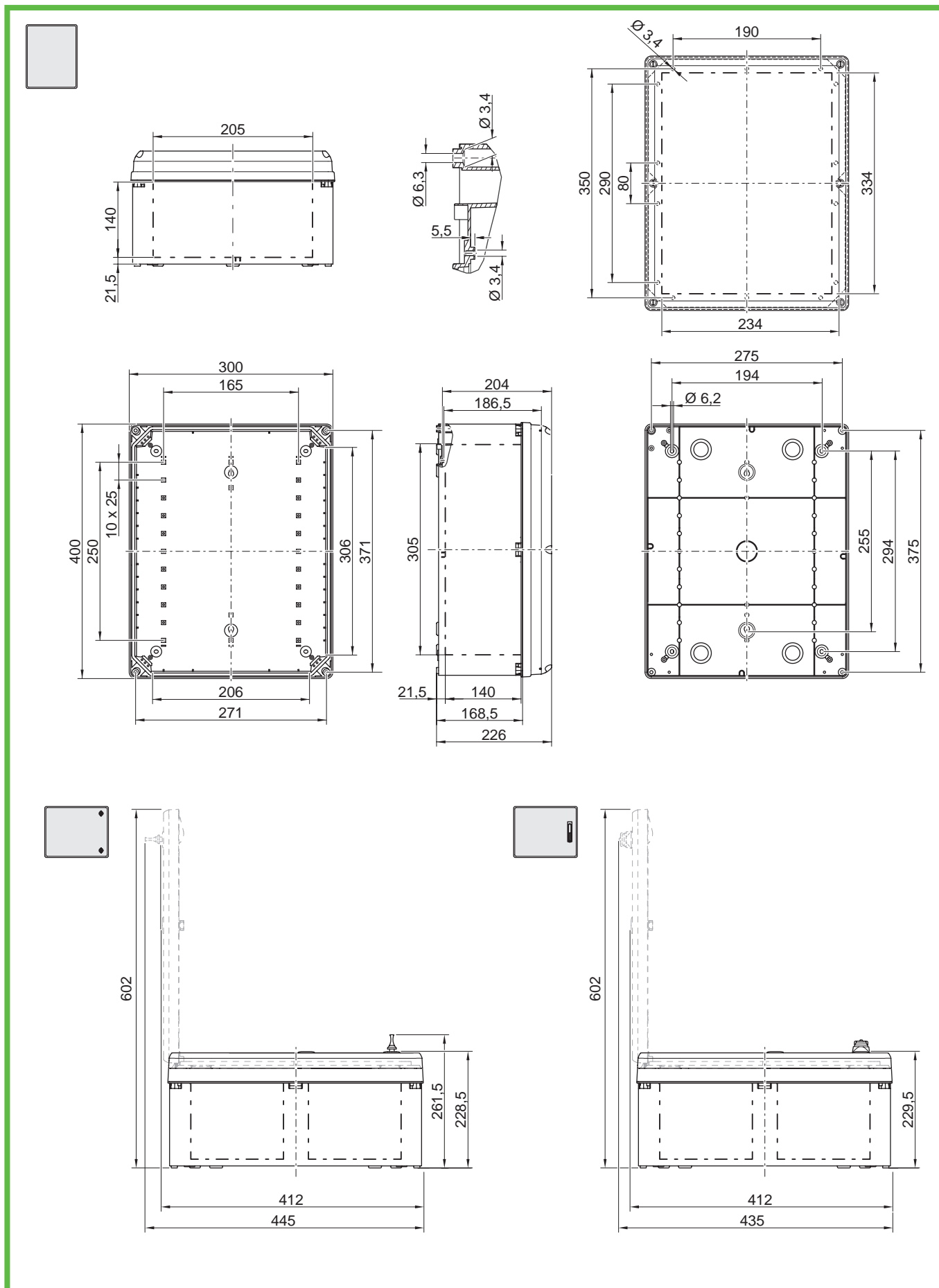
Abb. 95: GEOS-S 4030-22
