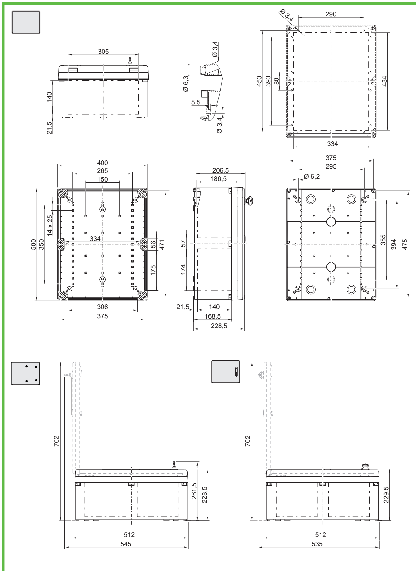
Abb. 97: GEOS-S 5040-22
