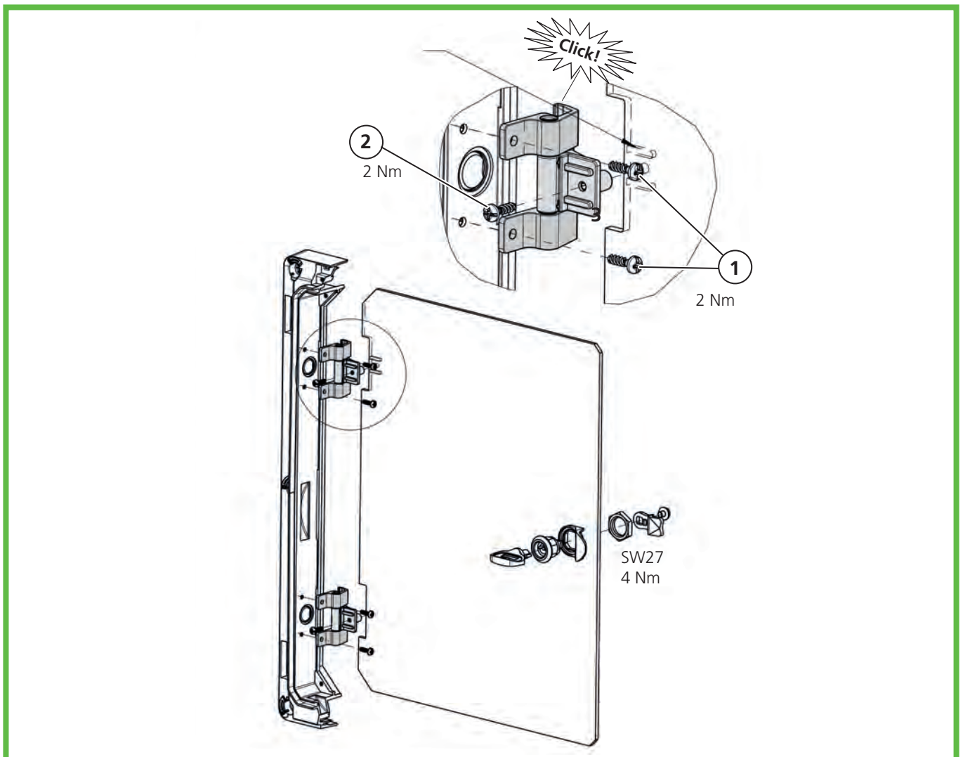
Abb. 87: Montage der Innentür
