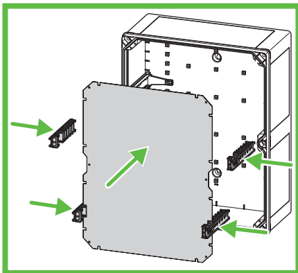
Abb. 73: Montage Montageträger in die Basisträger
