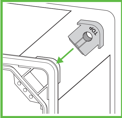
Abb. 49: Montage Gewindeinschübe GEOS 3030, GEOS 3040 GEOS 4050
