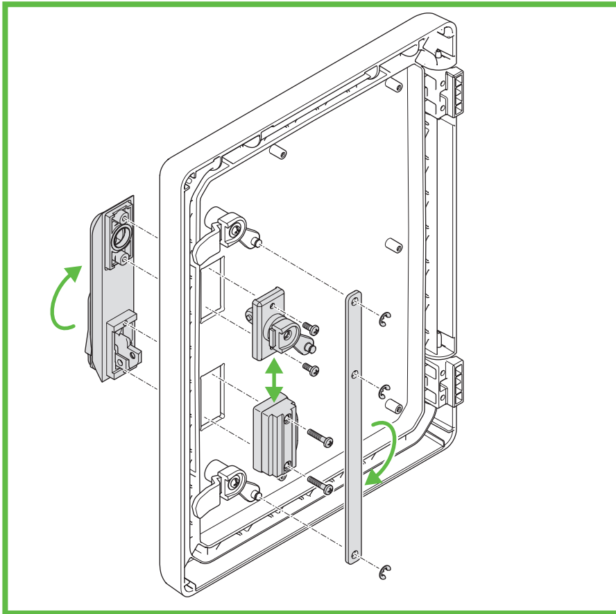
Abb. 66: Wechsel des Türanschlages bei Varianten mit Schwenkhebel
