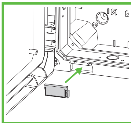
Abb. 61: Montage der Tür
