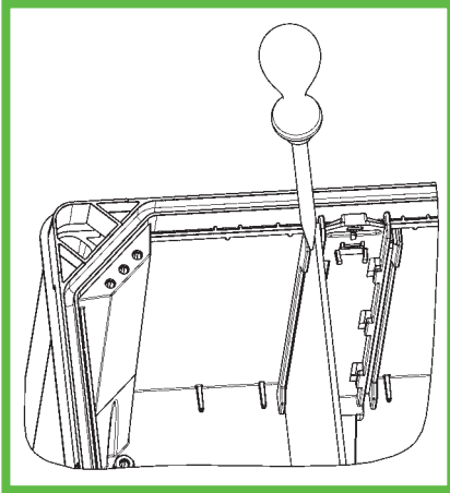
Abb. 86: Demontage Trennwand
