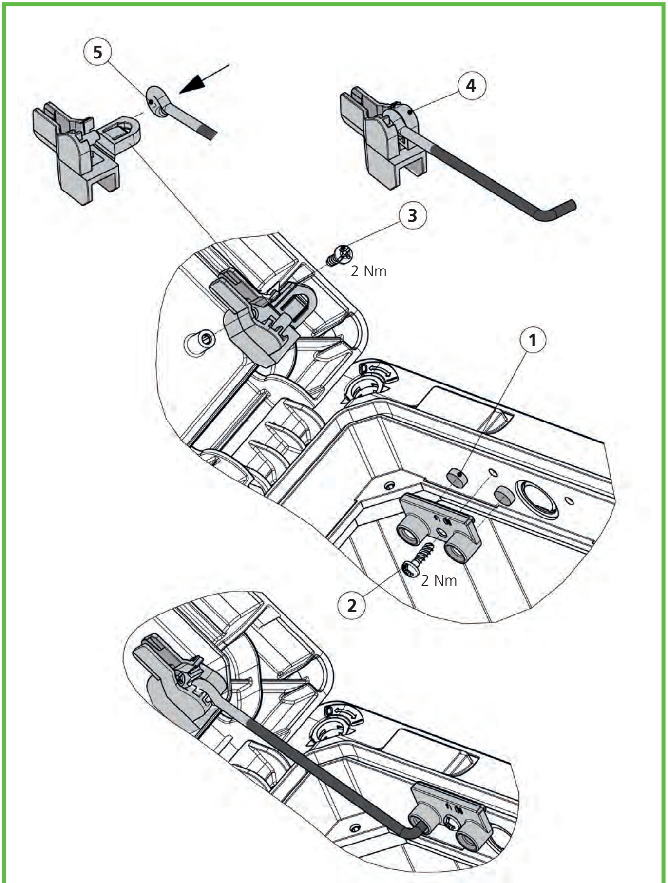
Abb. 88: Montage des Türaufstellers
