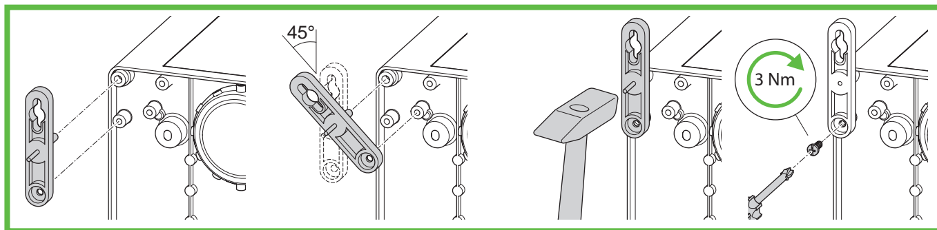
Abb. 43: Montage Außenbefestigungslasche ABL-10
