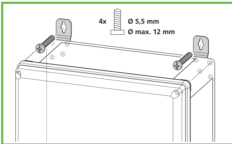
Abb. 47: Wandmontage
