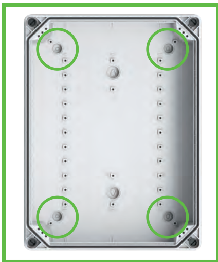
Abb. 40: Befestigungspunkte 4-Punkt-Montage
