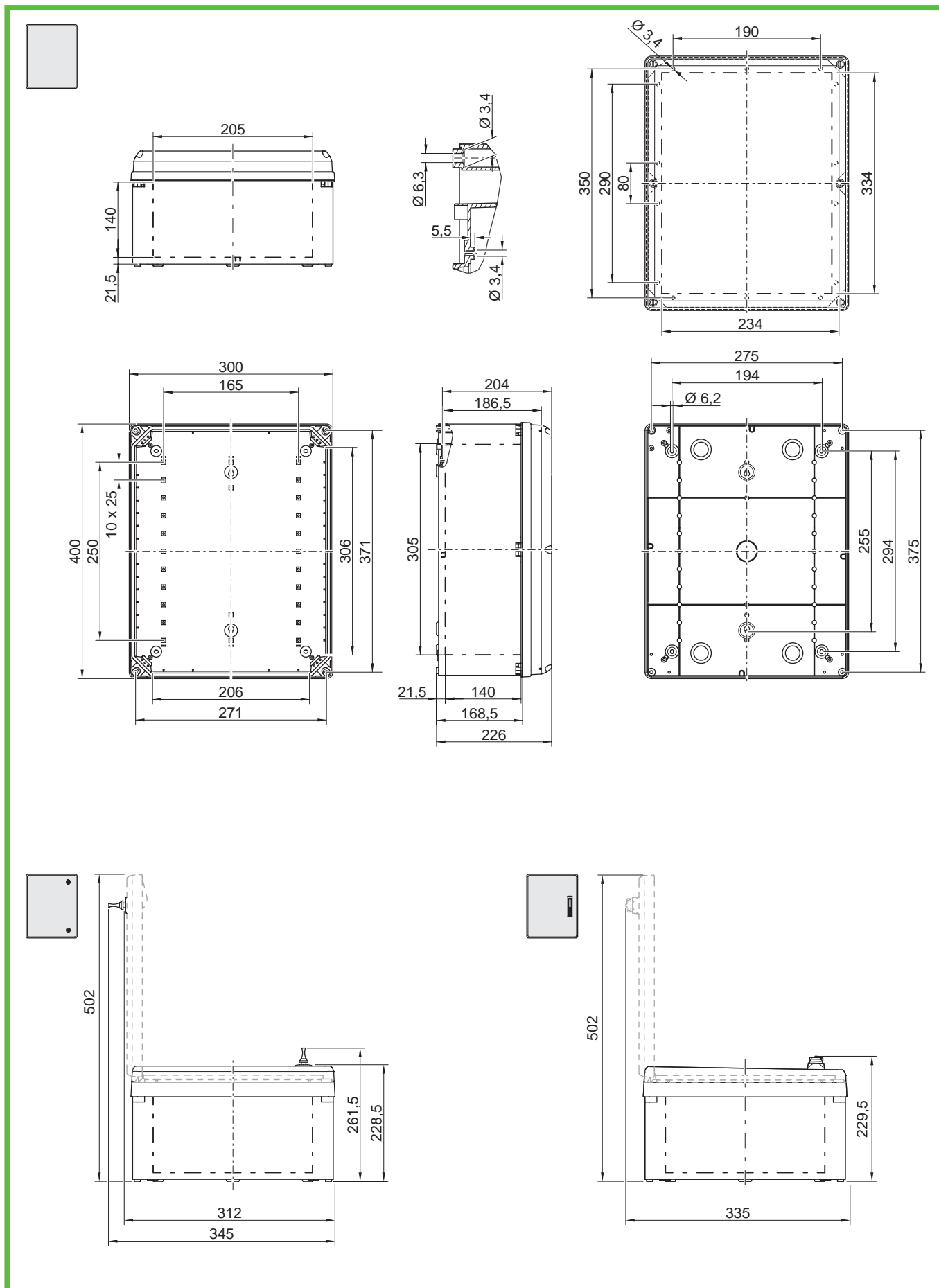
Abb. 93: GEOS 3040-22
