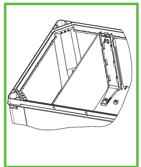
Abb. 85: Montierte Trennwand
