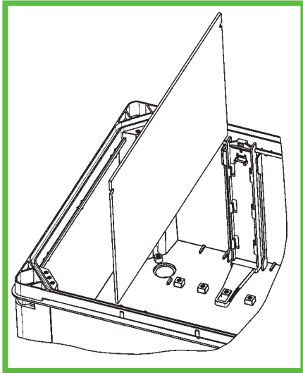
Abb. 78: Montage Trennwand
