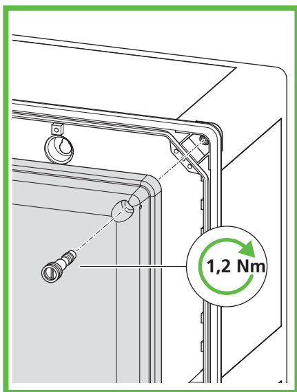
Abb. 53: Montage Schnellgewindeschraube
