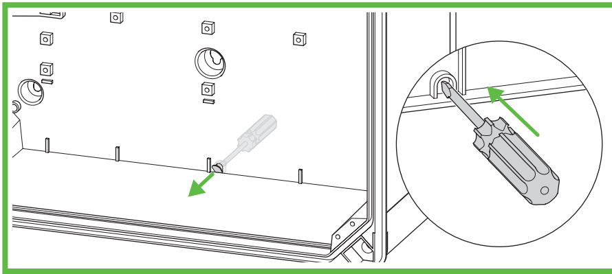
Abb. 39: Entwässerungsöffnung
