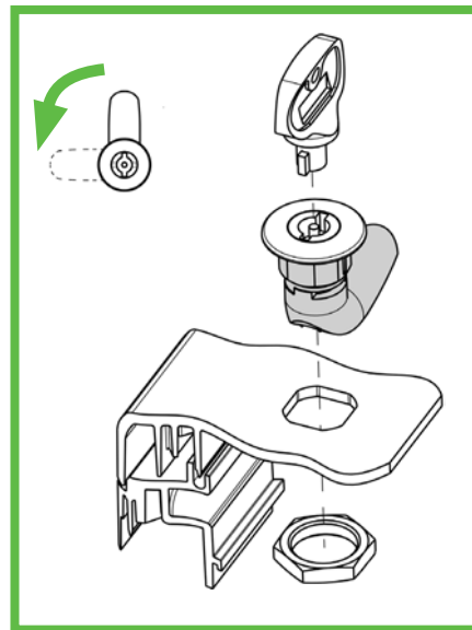
Abb. 64: Schließrichtung nach rechts
