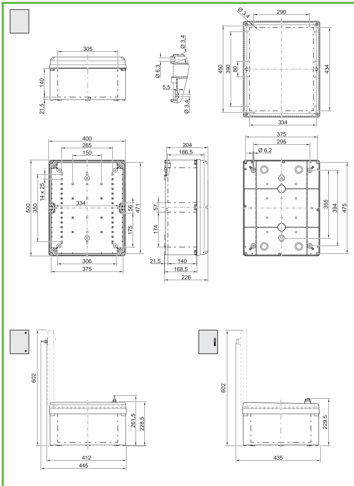
Abb. 96: GEOS 4050-22
