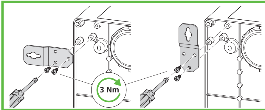
Abb. 46: Montage Außenbefestigungsflasche ABL-10/ES
