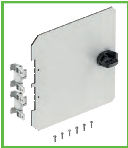
Abb. 34: Innentür mit Befestigungsmaterial
