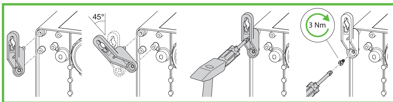
Abb. 44: Montage Außenbefestigungslasche ABL-40
