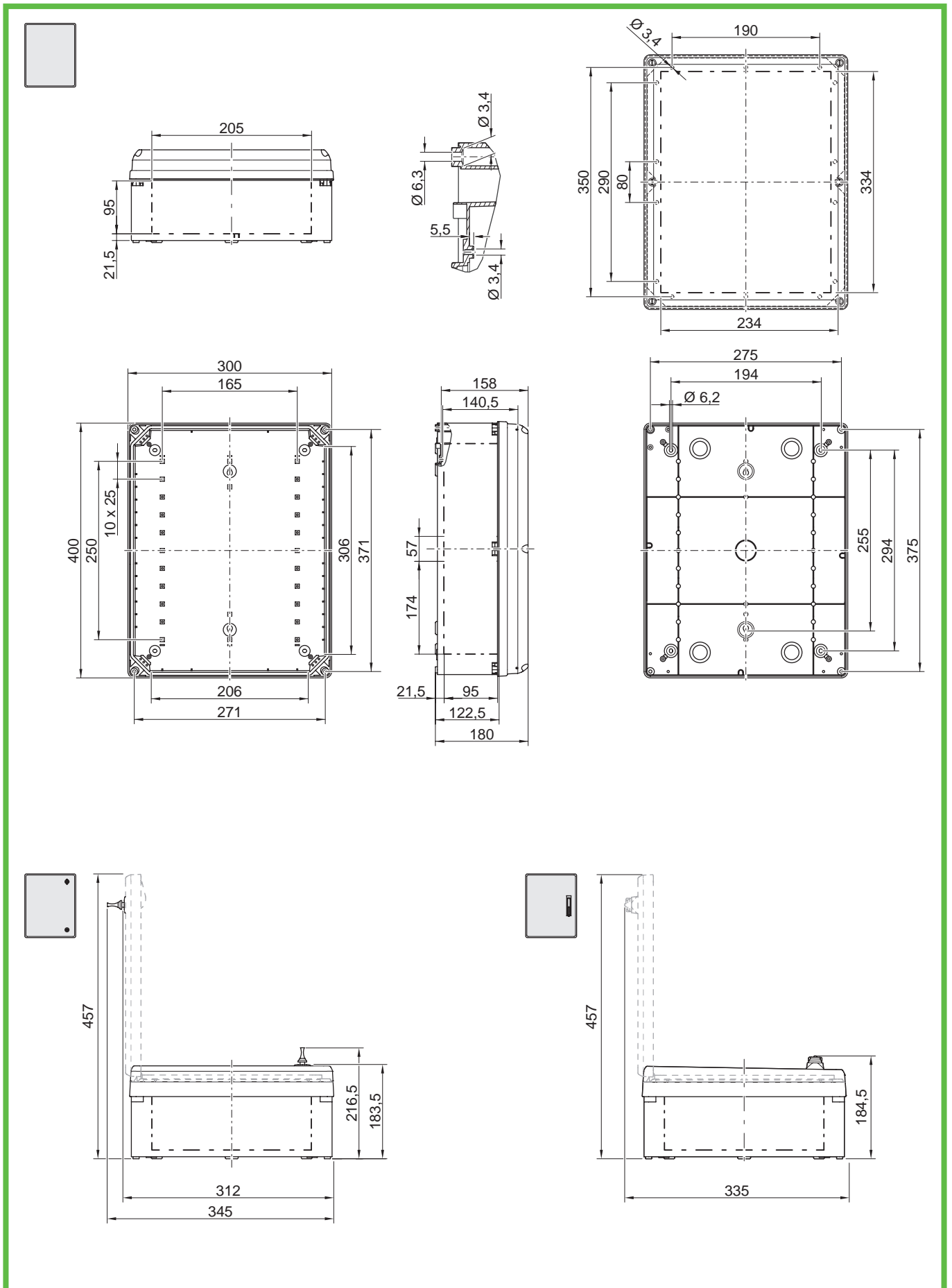
Abb. 92: GEOS 3040-18
