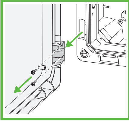
Abb. 63: Demontage der Tür
