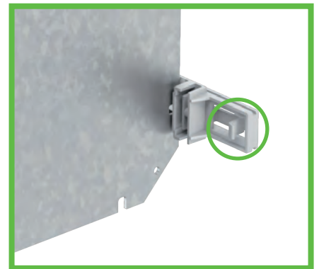
Abb. 69: Verriegelungshaken
