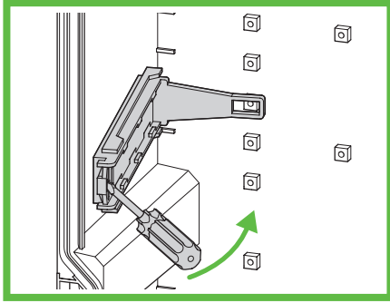
Abb. 72: Demontage Basisträger
