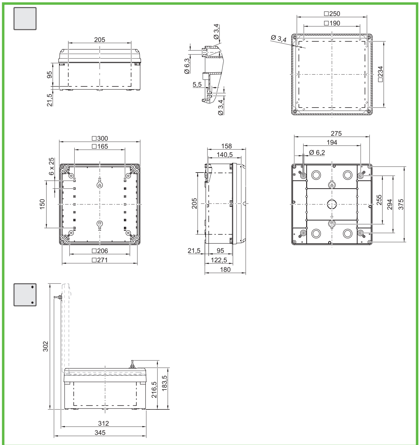
Abb. 90: GEOS 3030-18
