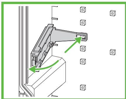
Abb. 70: Montage Basisträger
