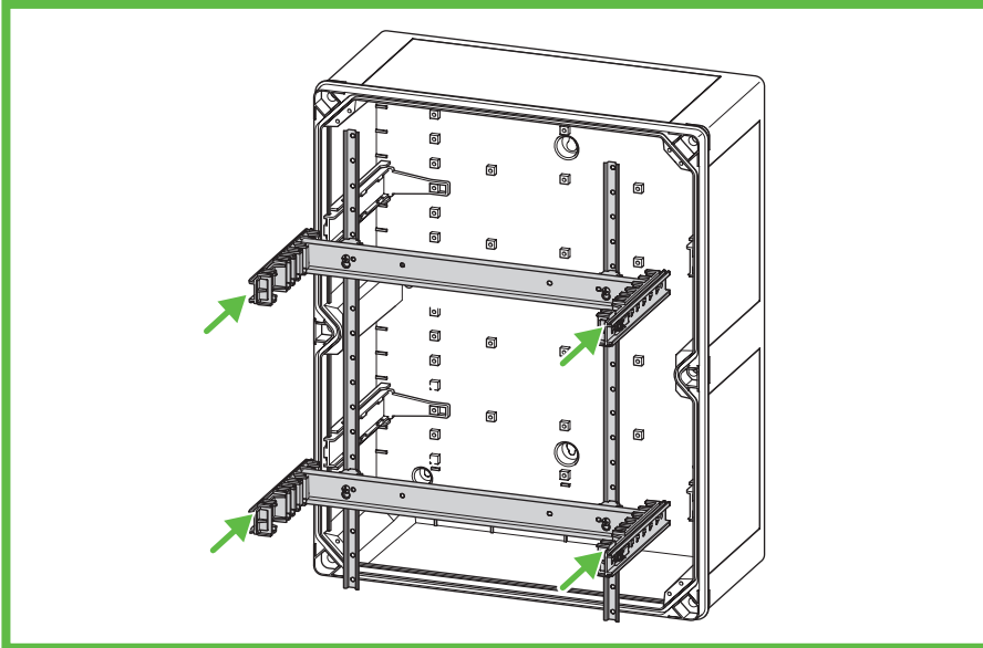
Abb. 76: Montage Traggestell in Kasten
