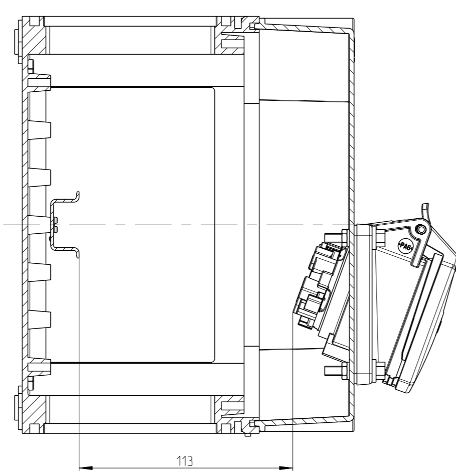
A-A
