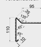
Abschlussprofil
