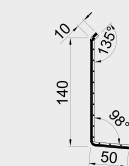
Wandanschluss
