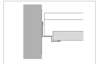
Nr. 50/14, Nr. 50/15 Contura-Decken System S 3a und System S 15a cliq
