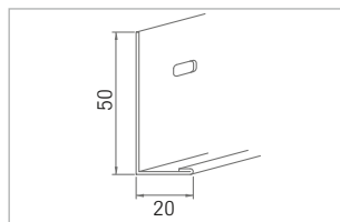
Nr. 51/20 1,0 mm dick
