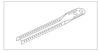
Nr. 16/... Abhänger-Verlängerung
