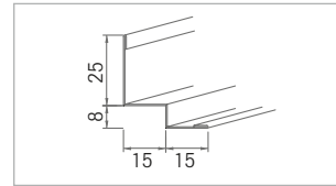
Nr. 50/15 0,5 mm dick
