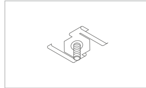
Nr. 95/30 (für 24 mm breite Schienen) Schraubklemme weiß
