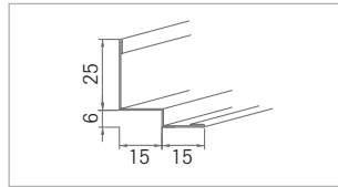
Nr. 50/14 0,5 mm dick
