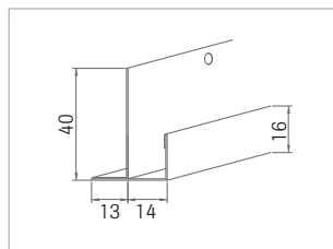
Nr. 8030/13 13er Platte 0,5 mm dick
