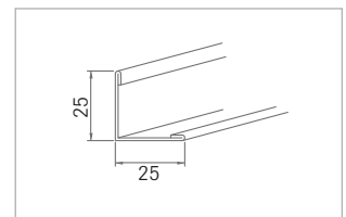
Nr. 51/25 1,0 mm dick
