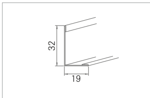
Nr. 51/32G 0,5 mm dick
