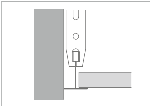
Nr. 45 o. cliq-24-MR Befestigung an der Rohdecke (gleitender Anschluss)
