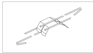
Nr. 12/.../1 bzw. Nr. 12/.../2* Schnellabhänger mit Doppelspannfeder doppelter Draht, vormontiert
