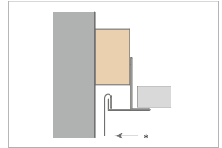
Nr. 8030/15 * = Befestigung für Dekorationen oder ähnliches. Für Punktlast bis max. 0,07 kN.
