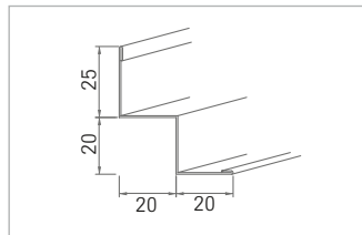
Nr. 56/20 0,6 mm dick Nr. 56/21 1,0 mm dick Nr. 56/23 1,5 mm dick
