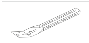
Nr. 17/80 Unterteil für Dreiecksaussteifungen
