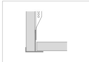
Nr. 8030/13, Nr. 8030/15 Deckenversprung oder Abschottung
