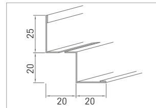
Nr. 56/35 0,6 mm dick (mit Lüftungsschlitzen)
