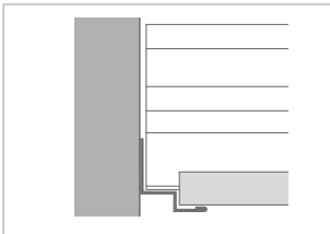
Nr. 50/22 freigesp. Decken, z. B. Flurdecken mit Contura-Platten nach System S 6b
