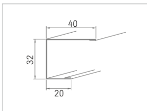
Nr. 57/10 0,6 mm dick
