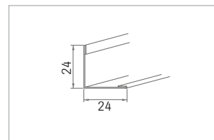
Nr. 51/24G 0,5 mm dick
