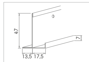
Nr. 8030/15 15er Platte 0,6 mm dick
