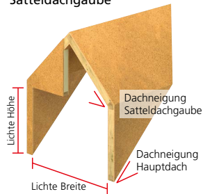
Satteldachgaube
