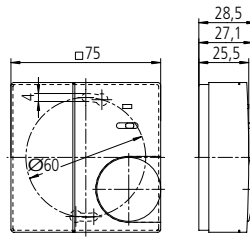
Raumsender, mit und ohne BA-Schalter
