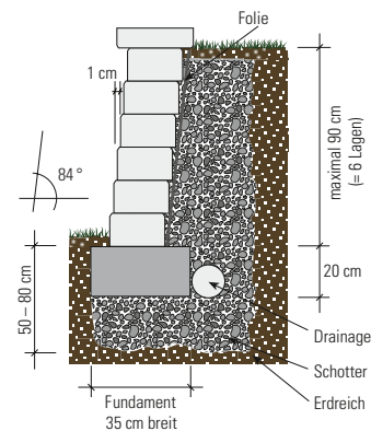
Aufbauminkel von 84°, hinterfüllt, mit Grundelement, ohne Verkehrslast
