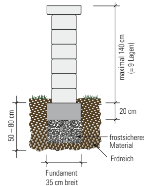
Freistehender Aufbau mit Grundelement
