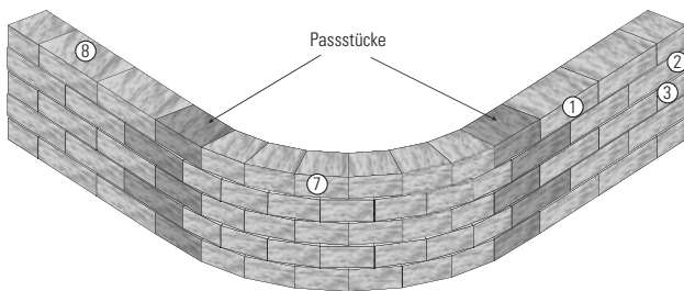
90°-Bogen mit bauseitig herzustellenden Passsteinen
