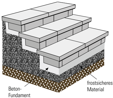
Einbau von Legestufen
