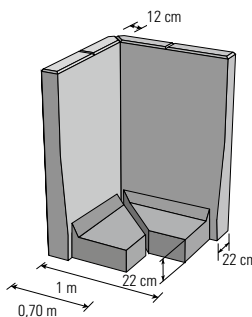
90°-Mauerscheiben-Außenecke, zweiteilig 12er SB-MS ab 1,80 m
