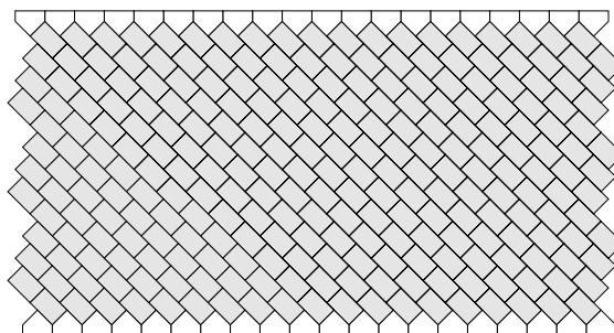
Geräuschkindernde Diagonalverlegung
