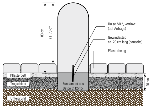
Einbaubeispiel MultiKegelpoller
