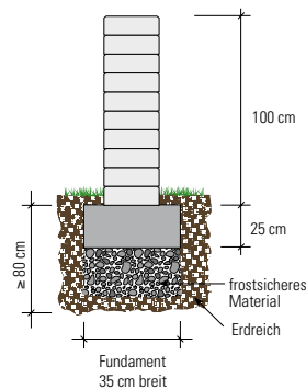
Freistehender Aufbau
