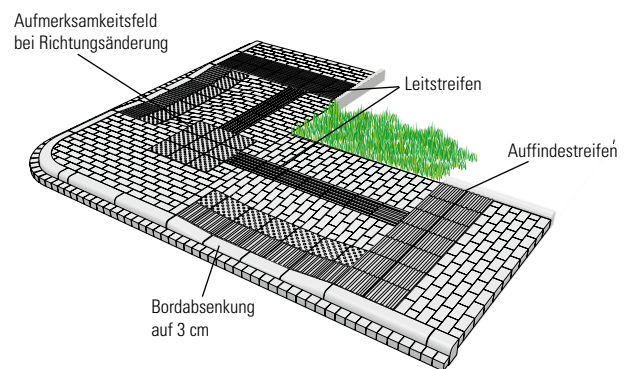
Abb. 25: Querung an einmündenden Straßen oder Kreuzungen bei nicht vorhandener oder gestörter, innerer Leitlinie
