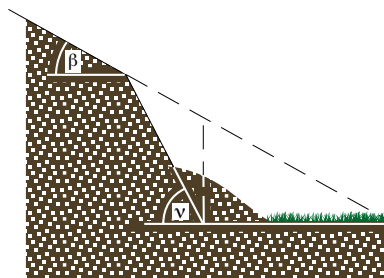
Senkrechte Abschachtung: Das Gelände rutscht nach.
