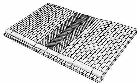
Abb. 27: Querung im Straßenverlauf
