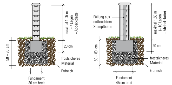
Freistehender Aufbau
