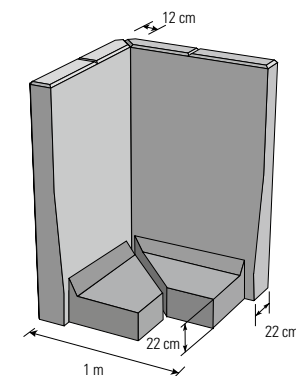
Mauerscheiben-Ecken Höhe 1,80 m–3,05 m
