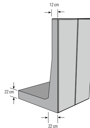
Mauerscheiben Höhe 1,80 m–3,05 m
