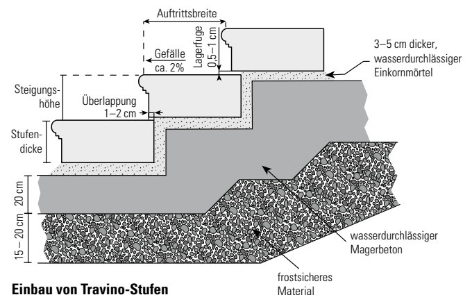
Einbau von Travino-Stufen
