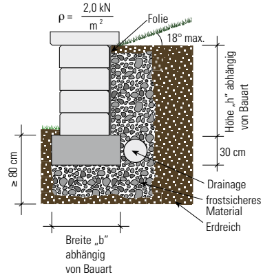
Senkrechter Aufbau, hinterfüllt mit Böschung
