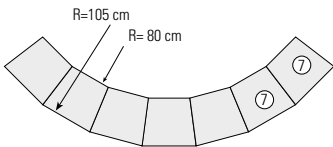
Radius bei Verwendung des Radiensteins
