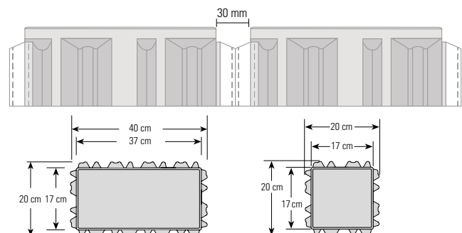
MultiTec-Öko mit KANNtec 10 -Verschiebeschutz für 30 mm breite Grünfuge.
