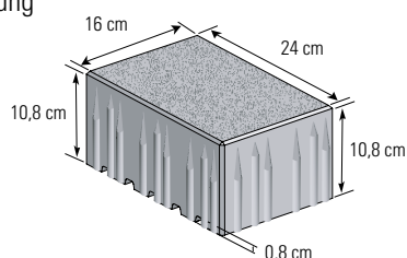
Planolith 5f, Verlegung im Splittbett
