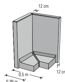
90°-Mauerscheiben-Außenecke, zweiteilig 12er SB, Vios-MS bis 1,55 m
