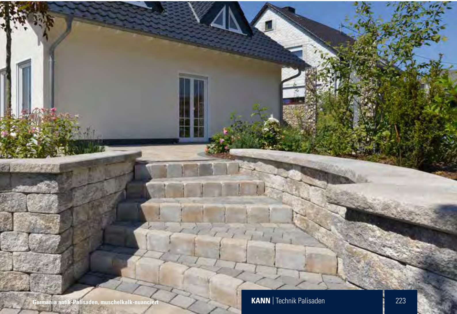
Einbau von Palisaden und Pflaster als Stellstufen
