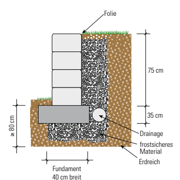
Senkrechter Aufbau, hinterfüllt, ohne Verkehrs-last
