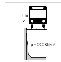
Lastfall 5b
