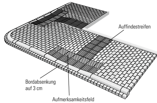
Abb. 24: Querung an einmündenden Straßen oder Kreuzungen
