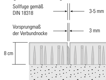
Der KANNtec-Verschiebeschutz vereinfacht das Herstellen einer normgerechten Fuge.
