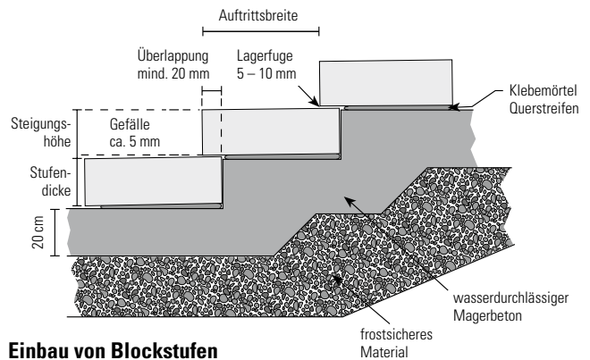
Einbau von Blockstufen
