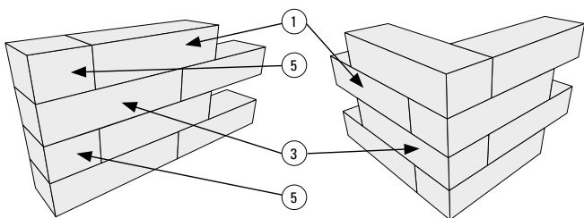
Aufbau der Vios-Mauer mit großformatigen Elementen (Drittelversatz)
