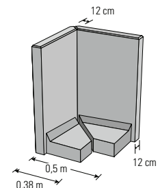
90°-Mauerscheiben-Außenecke, zweiteilig 12er SB, Vios-MS bis 1,55 m
