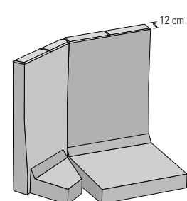
135°-Mauerscheiben-Außenecke, zweiteilig (aus Eck- und Normalelement) 12er SB-MS
