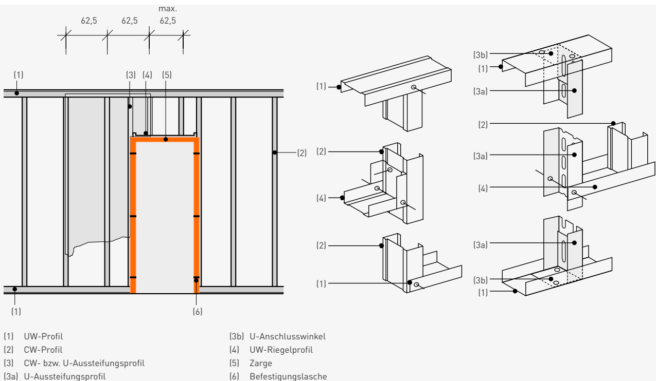
Einbauschema der Zarge mit Unterkonstruktion
