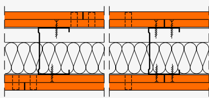
Montagewand mit fermacell® Gipsfaserplatten als Einfachständerwand, doppellagig bekleidet. Äußere Plattenlagen in 1./untere Plattenlagen geklammert
