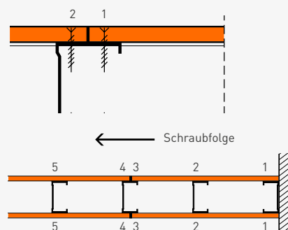
Anordnung der Plattenstöße bei einlagiger fermacell® Bekleidung
