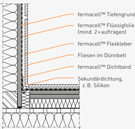
Boden-Wand-Anschluss
