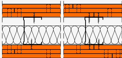
Montagewand mit fermacell® Gipsfaserplatten mit Hohlraumdämmung als Einfachständerwand, dreilagig bekleidet. 2.+3. Plattenlage in 1. untere Plattenlage geklammert
