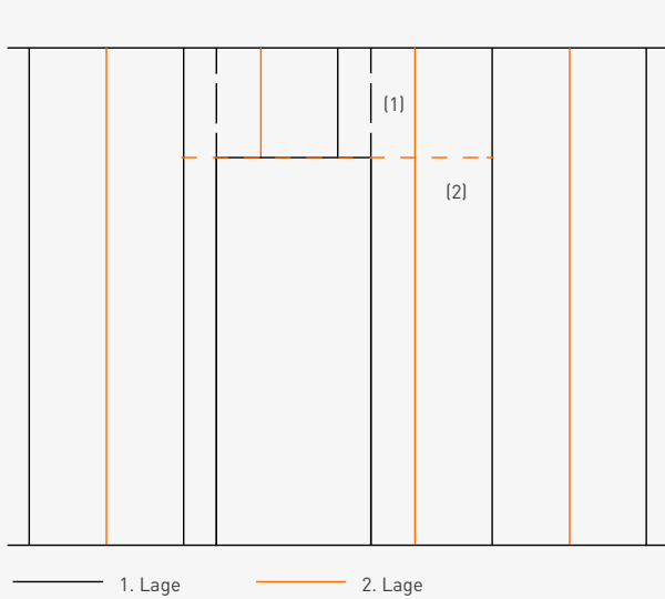
Bekleidungschema zweilagig bekleidete Montagewand mit fermacell® Gipsfaserplatten
