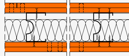
Hoch schalldämmende Montagewand mit fermacell® Gipsfaserplatten, doppellagig bekleidet
