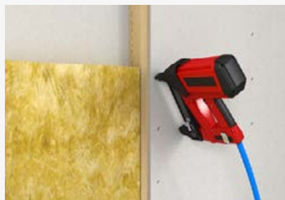
Klammern auf Holzunterkonstruktion
