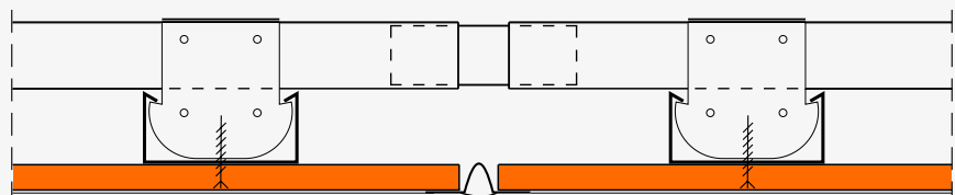
Decken-/Dachkonstruktion mit fermacell® Gipsfaserplatten ohne Brandschutzanforderung. Bewegungsfuge mit Zusatzprofil.
