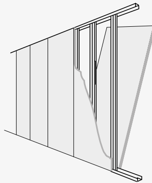
Aufstellen einer Montagewand mit fermacell® Gipsfaserplatten
