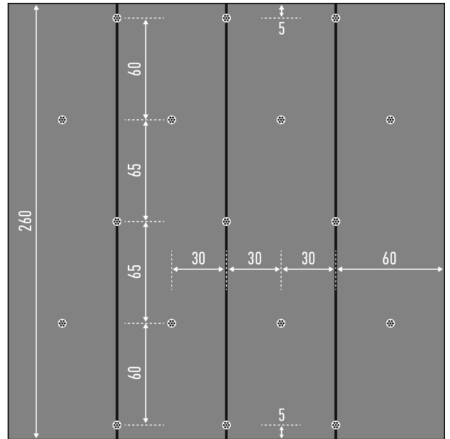
Bei vollflächiger Verklebung auf den Untergrund: Sopro Board ab 4 mm Dicke
