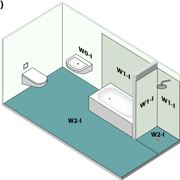
Häusliches Bad mit Badewanne und bodengleicher Dusche.
