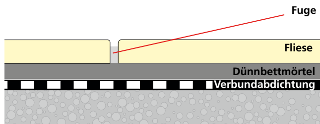
System: Fliesenverbundabdichtung.
