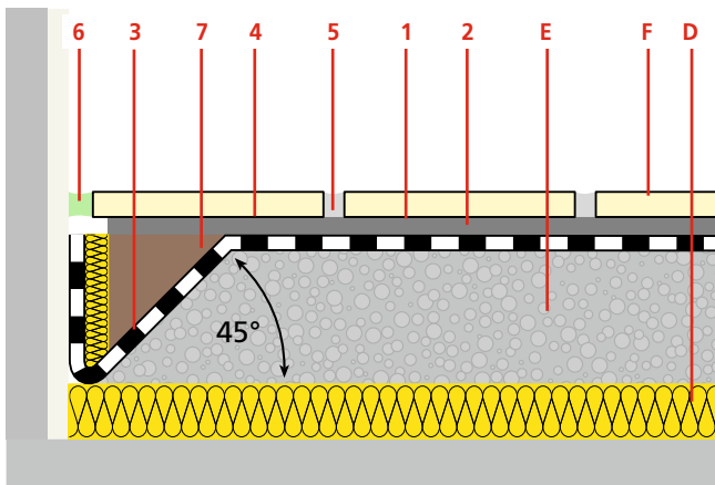
Die Wandfläche innerhalb des Estrichquerschnittes wird als Klebefläche zur Anbindung der Verbundabdichtung verwendet.
