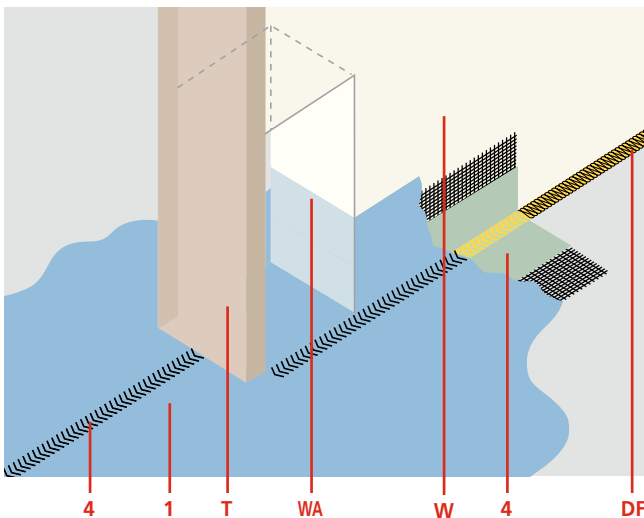
Lösung bei vorhandener Türzarge.
