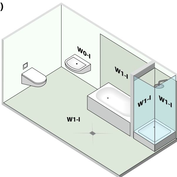
Häusliches Bad mit Badewanne und Duschtasse mit Duschtrennung: Bodenablauf im Raum.
