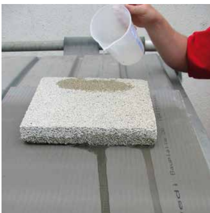
Leichter Wasserabfluss in einer Drainageestrich-Musterplatte.
