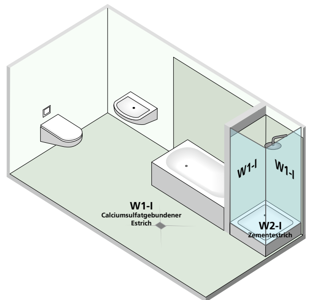
Bad mit wirksamem Spritzwasserschutz im barrierefreien Duschbereich.
