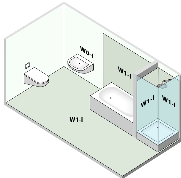
Häusliches Bad mit Badewanne und Duschtasse mit Duschatrennung.
