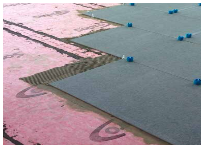
12 Einlegen der Platten in das vorbereitete Mörtelbett.
