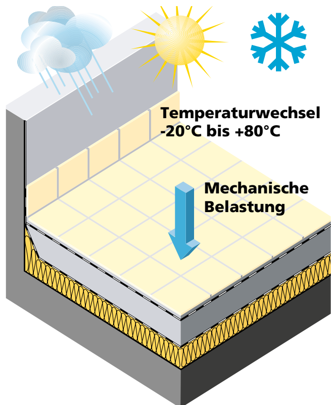
Balkon/Terrasse (über bewohntem Raum) mit den entsprechenden Belastungen.
