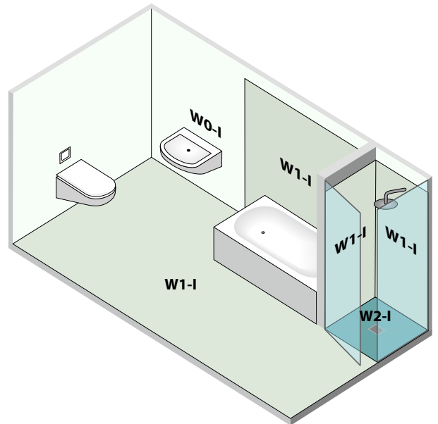
Häusliches Bad mit Badewanne und bodengleicher Dusche mit Duschtrennung.
