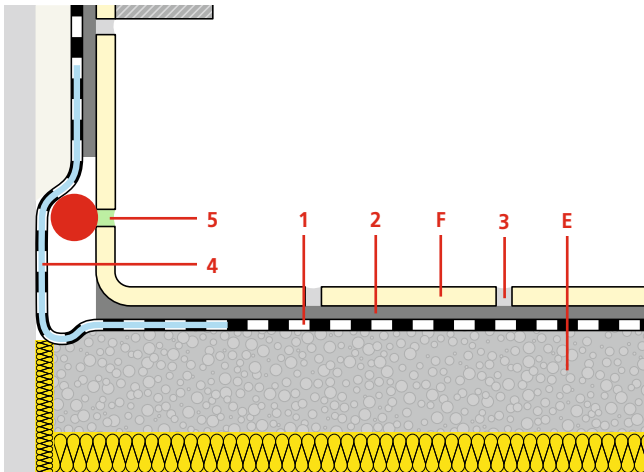
Hohlkehlsockelanschluss mit Verbundabdichtung.
