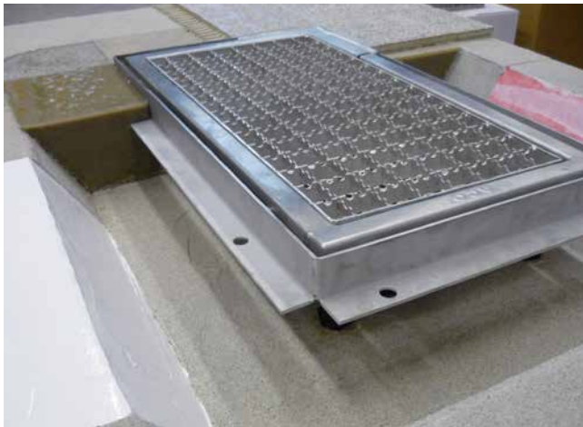
Schnitt durch eine Rinnenmulde. Sehr gut ist der umlaufende Edelstahlrahmen zu erkennen, der zusätzlich als Kantenschutz für die anliegenden Fliesen dient.
