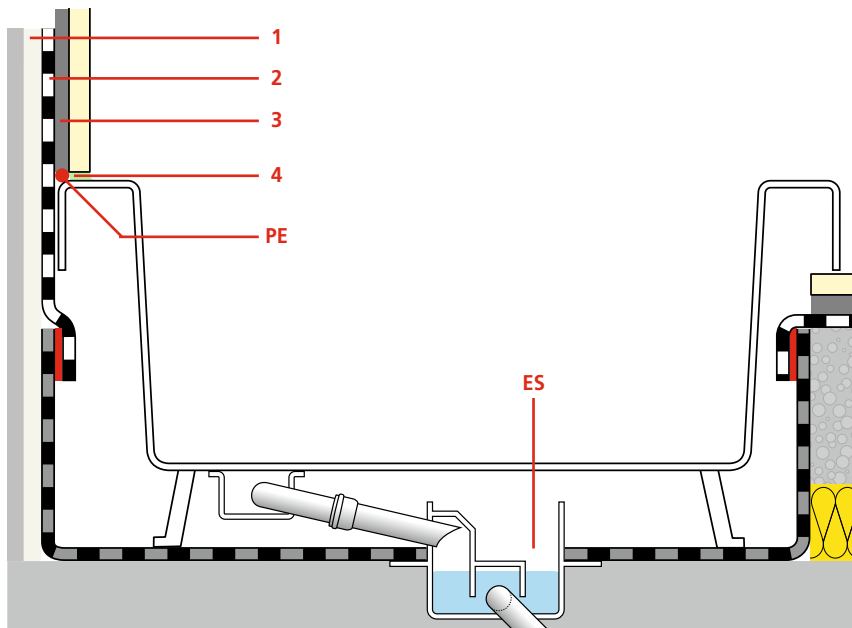
Entwässerungstopf zur Zwischenentwässerung einer Abdichtungsebene.
