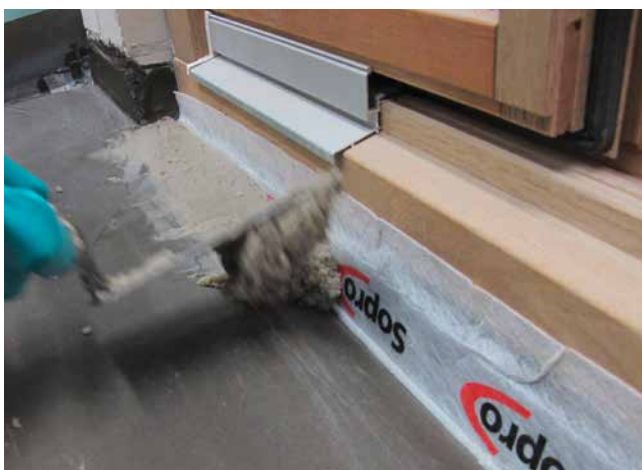
5 Nach dem Einstellen eines Randdämmstreifens wird die Vertiefung mit einem schwindarmen und kapillardichten Reaktionsharzmörtel verfüllt.
