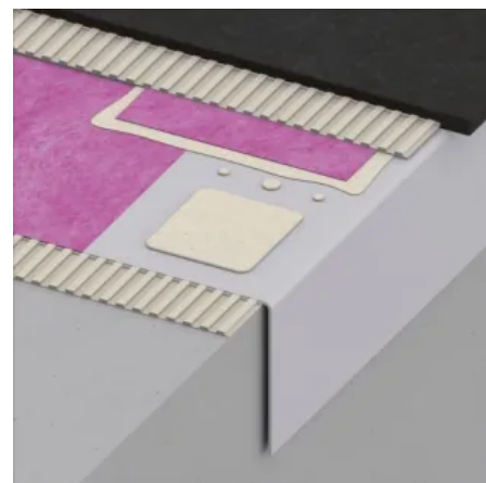
alferbal Balkonwinkel-Profil
