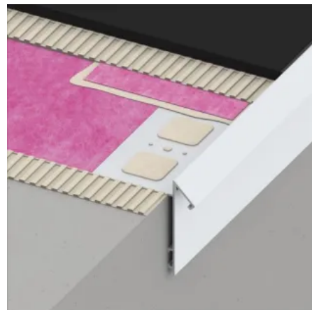
alferbal Tropfkanten-Profil
