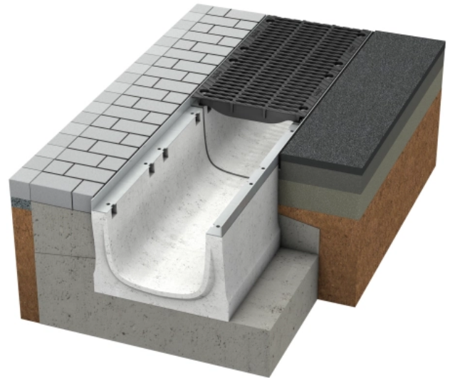
BIRCOsir® Entwässerungsrinnen mit großen Retentionsraum
