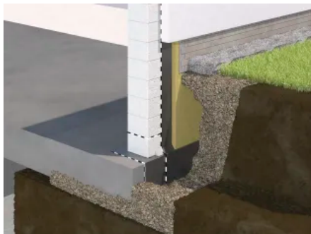
Kelleraußenwand
