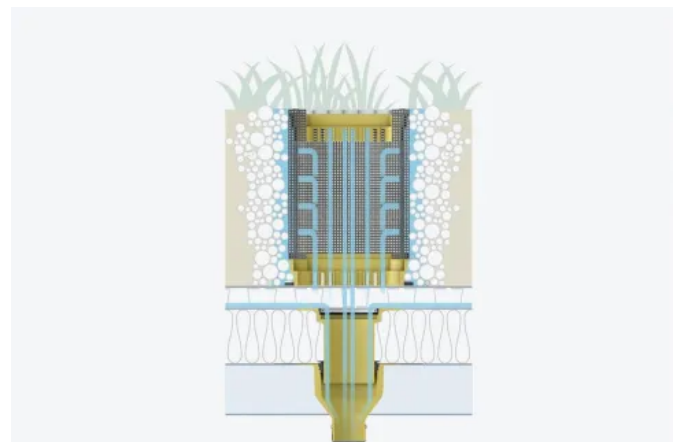
D. Für extensive und intensive Dachbegrünung: SitaGreen Gründachschacht
