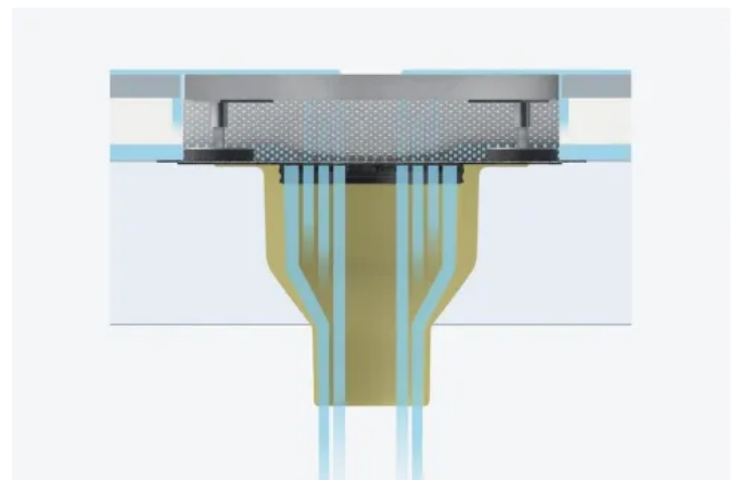
E. Mit Gitterrost zur Terrassenentwässerung: SitaDrain Terra
