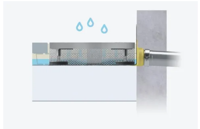
A. Mit optimal höhenverstellbaren Füßen: SitaDrain® Terra
