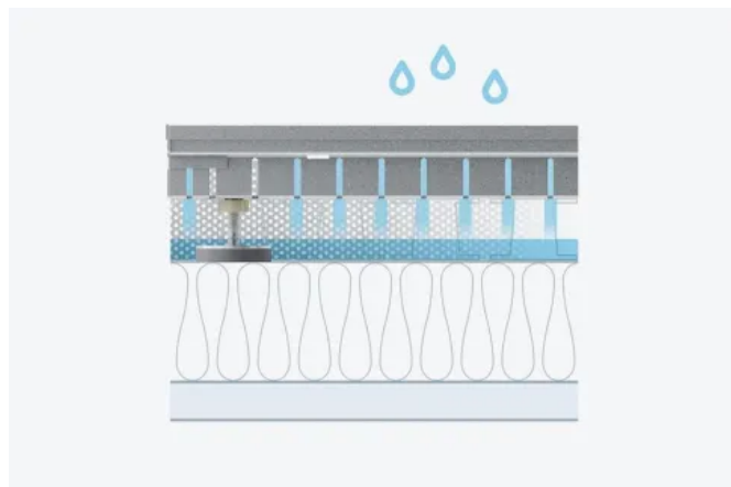
B. Mit Kiesleiste: SitaDrain® Kastenrinne
