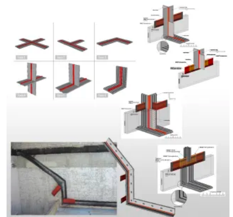
Systemfugenbänder
