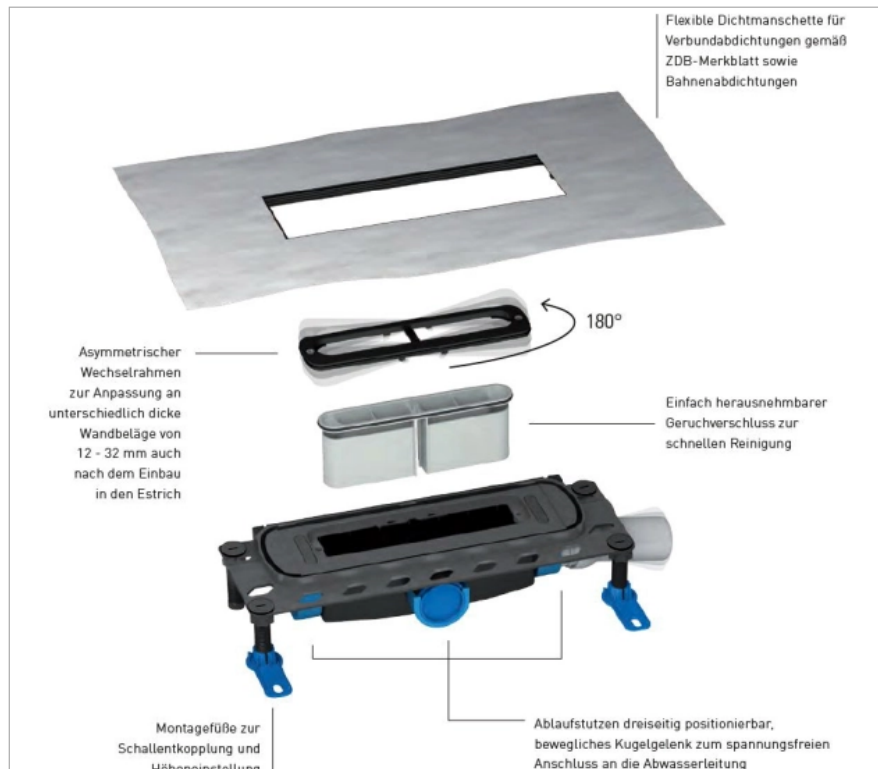
Ablaufgehäuse DallFlex
