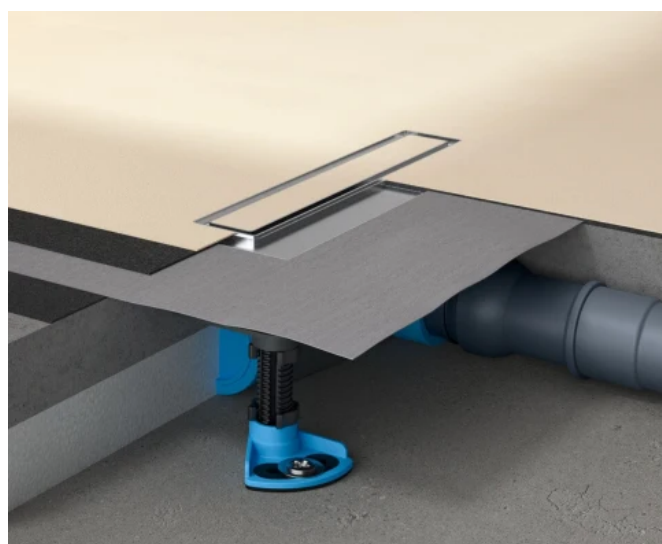
Duschrinnen CeraFrame Liquid waagerecht
