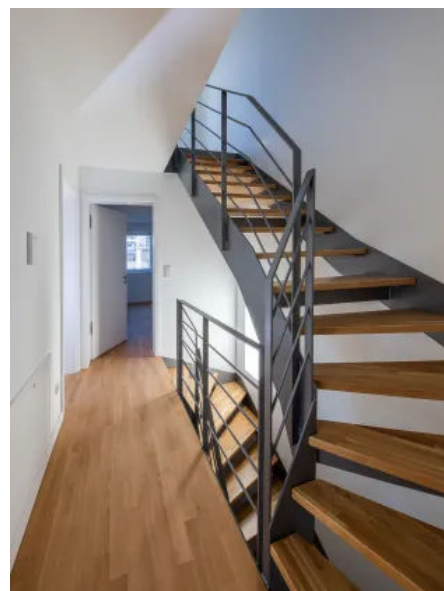
Flachstahlwangentreppe
