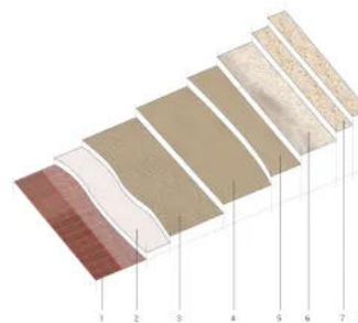
LIXIO®-Mikroterrazzo – Systemaufbau
