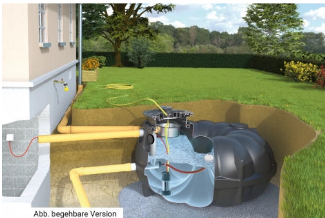
Garten-Kompletanlage Retention und Nutzung – Regenwassernutzung kombiniert mit Rückhaltung mit Wasseranschluss im Tankdeckel
