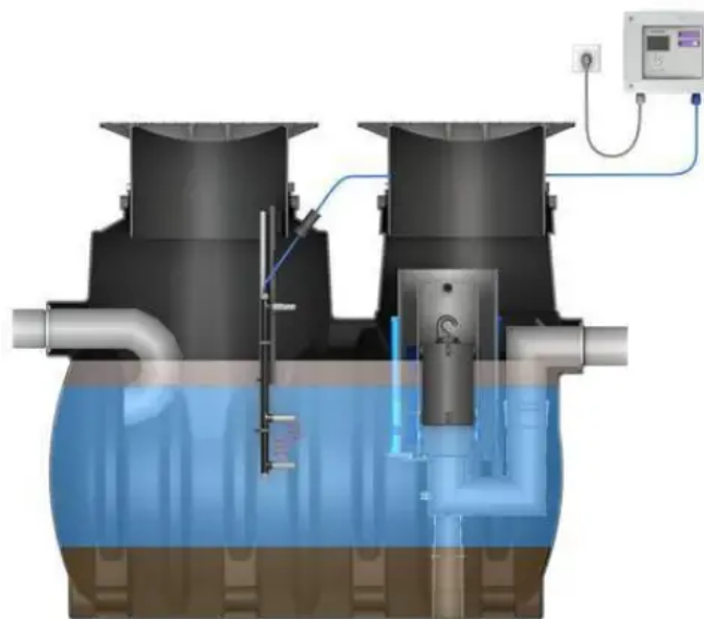
Funktionsprinzip SonicControl
