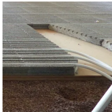
LITHOWOOD: Aufbau im Querschnitt
