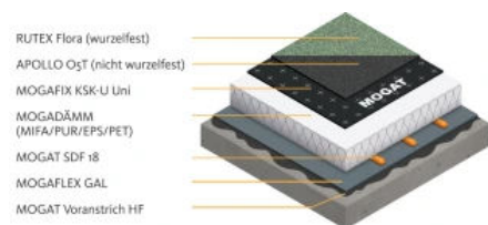
Neudach auf Beton
