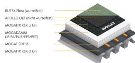
Neudach auf Trapezblech
