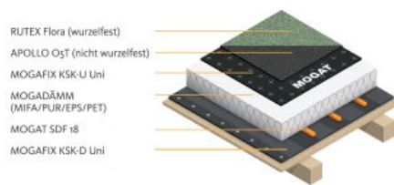
Neudach auf Holz
