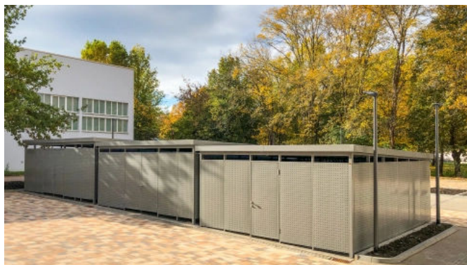
Mülltonnen-Einhausung geschlossen, Modulbauweise, Quadratlochblech
