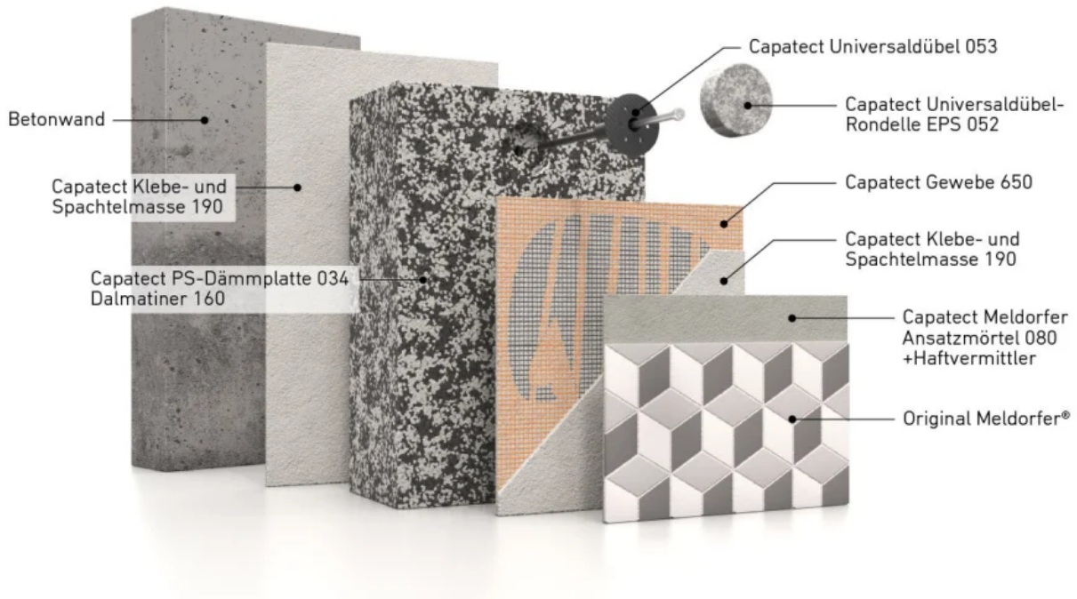
Beispielhafter Systembau mit Original Meldorfer®
