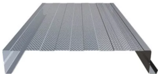
Kassette SAB B90/500, Beschichtung Colorcoat Prisma SV Blank RAL 9003 Signalweiß
