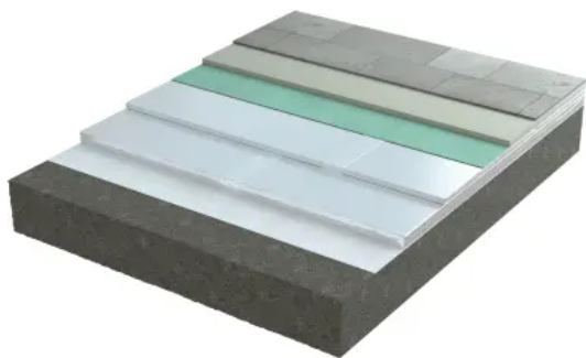
Bodenaufbau mit Promat ULTIMA® VIP
