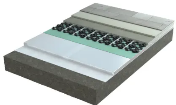
Bodenaufbau mit Promat ULTIMA® VIP unter einer Fußbodenheizung
