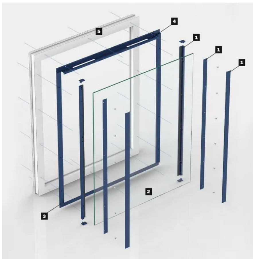
Systemaufbau
