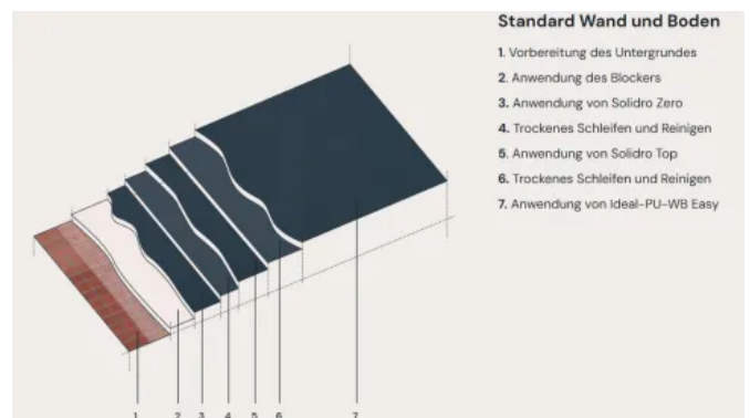
Solidro – Systemaufbau 1, Wand und Boden
