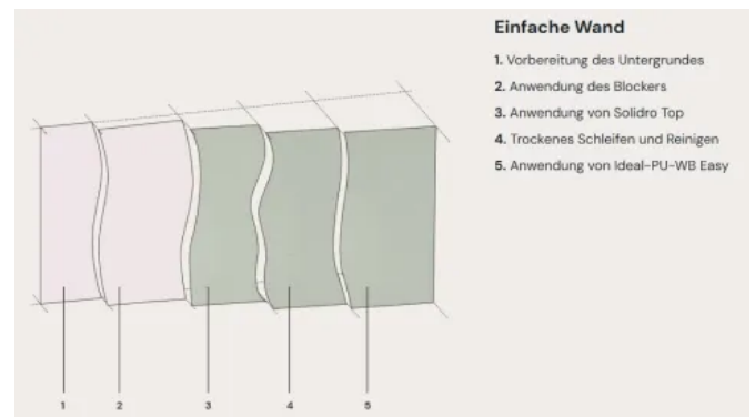
Solidro - Systemaufbau 3, Wand
