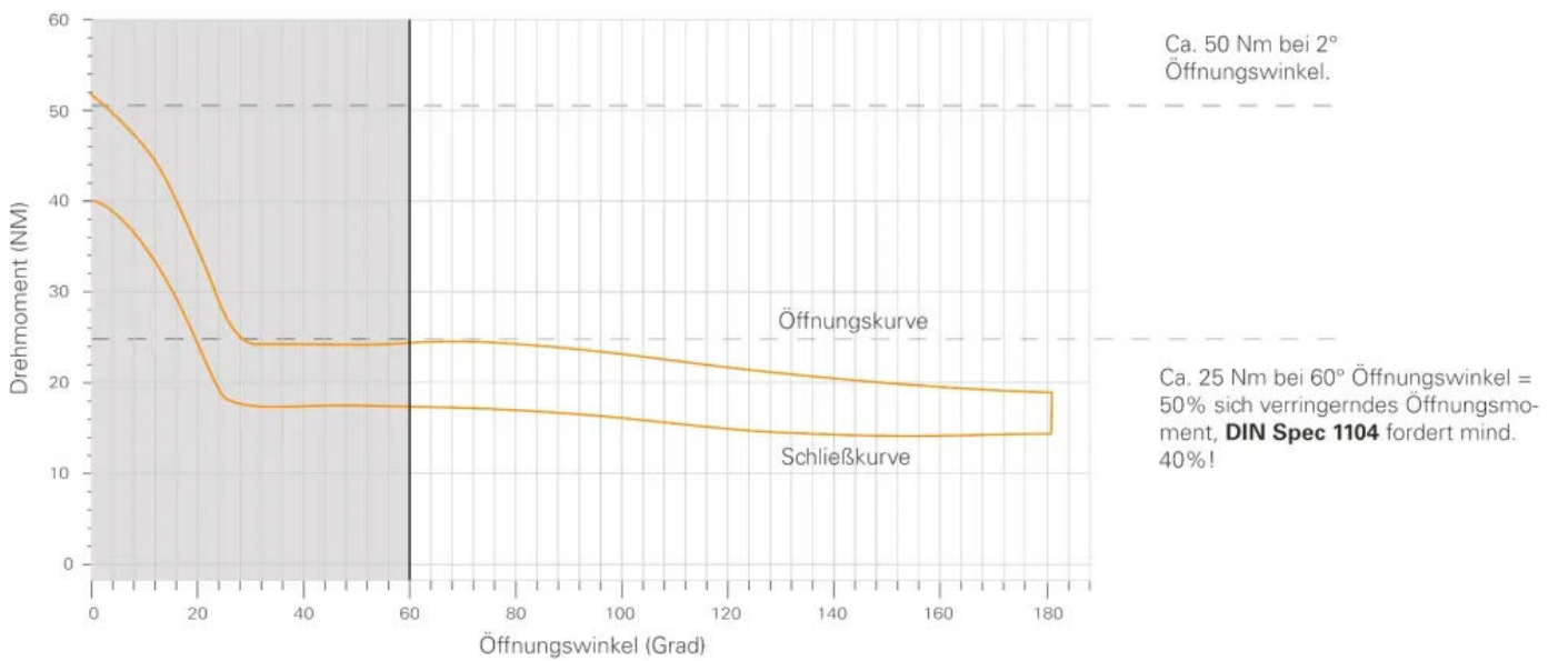
Drehmomentenverlauf Obentürschließer GTS 640
