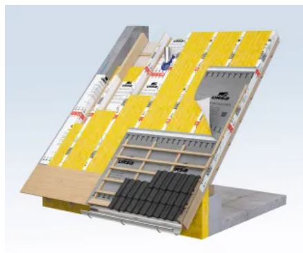
URSA Zwischensparrendämmung von außen
