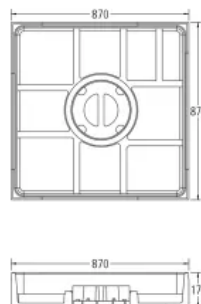
Poresta® Compact 2 Duschwannenträger 2.0 für quadratische und rechteckige Duschwannen aus Stahl oder Acryl
