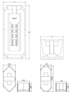
Poresta® Compact, Badewannenträger Ausführung Rechteck, Sechseck, Achteck, Oval
