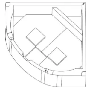
Poresta® Badewannenträger ohne Ablage für Eckwanne (Wannenrand bündig)
