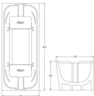
Poresta® Vario, Badewannenträger für eine senkrechte oder schräge Ausführung der Seiten
