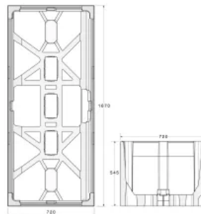
Poresta® Compact 2 Badewannenträger mit 2 senkrechten Längsseiten und 3 Ablaufbereichen zum variablen Einbau
