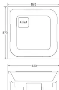
Poresta® Duschwannenträger für Duschen aus Stahl oder Acryl
