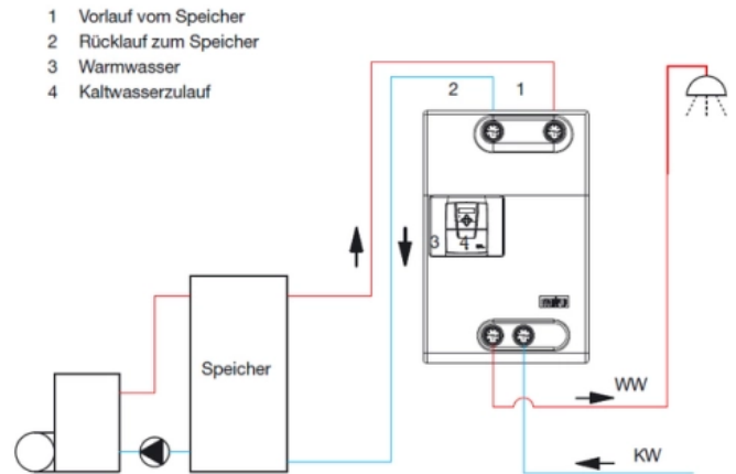
Schaltschema
